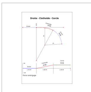
Raccordement par clothoïde.svg 512 × 723; 77 KB
