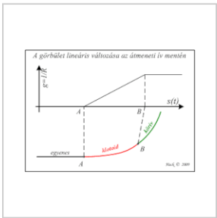
Átmeneti ív csatlakozása.gif 304 × 217; 6 KB
